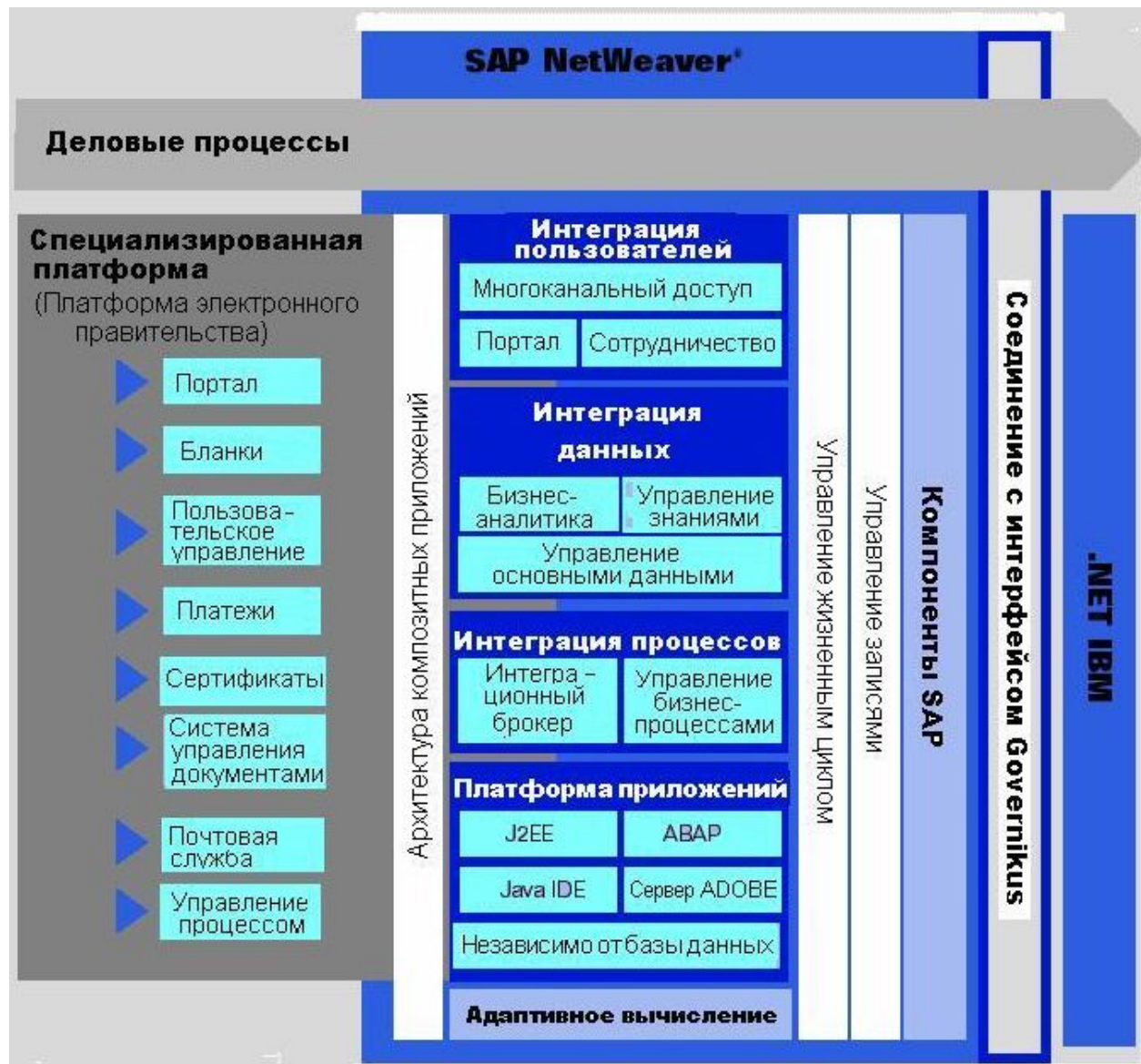
Открытая интеграционная платформа э-правительства для проекта BundOnline 2005, ФРГ.
